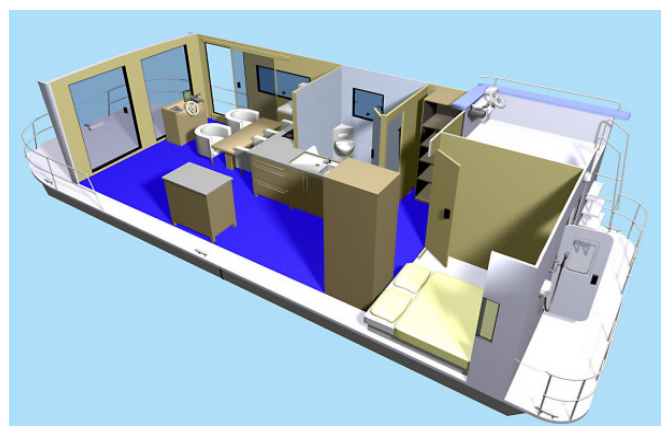
Innenraum / Layout SEADES 39 TA
